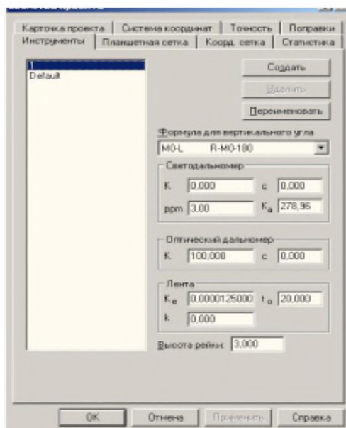
Рис. 5. Свойства проекта
