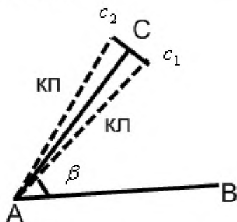
Рис. 10. Вынос в натуру проектного горизонтального угла
