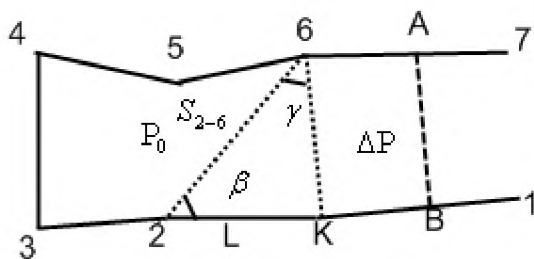
Рис. 8. Проектирование участка линиями, параллельной заданному направлению
