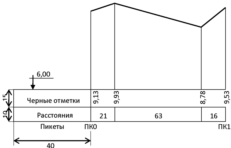
Рис. 10. Продольный профиль трассы
