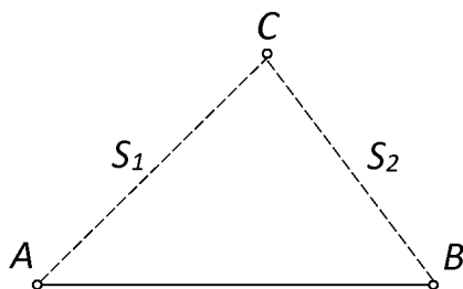
Рис. 4. Восстановление утраченного межевого знака способом прямой линейной засечки
