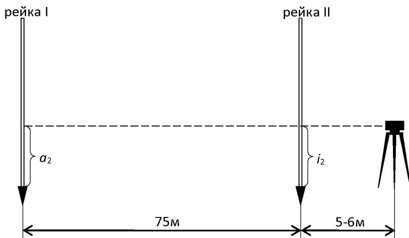
Рис. 7. Выполнение главной поверки нивелира а – установка нивелира относительно рейки I; б – установка нивелира относительно рейки II
