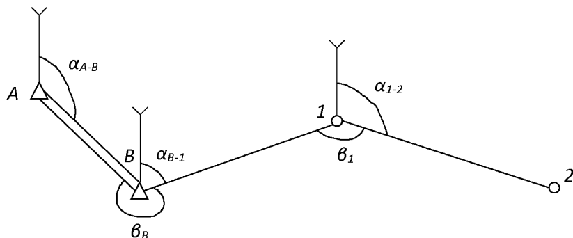
Рис. 4. Привязка съемочного обоснования к пунктам ГГС
