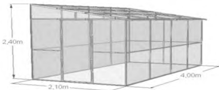
Рис. 6. Односкатная теплица
