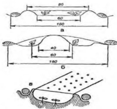
Рис. 4. Бескаркасный тип укрытия:
