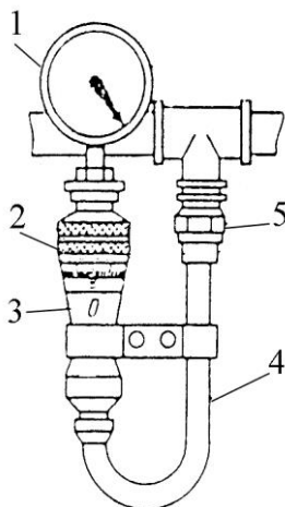
Рис. 7. Устройство индикатора КИ-4840:
