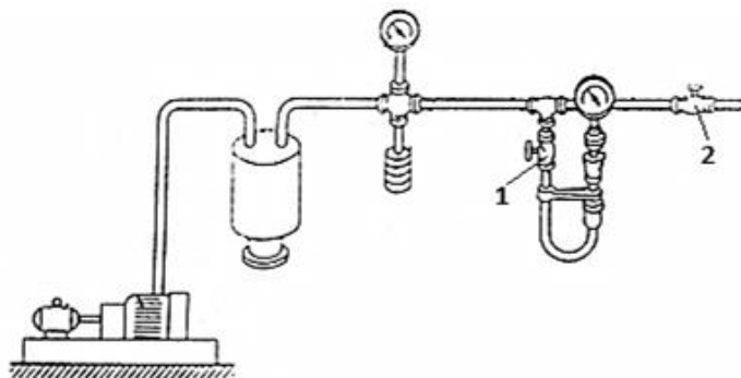
Рис. 8. Схема установки для определения подачи вакуум-насоса:
