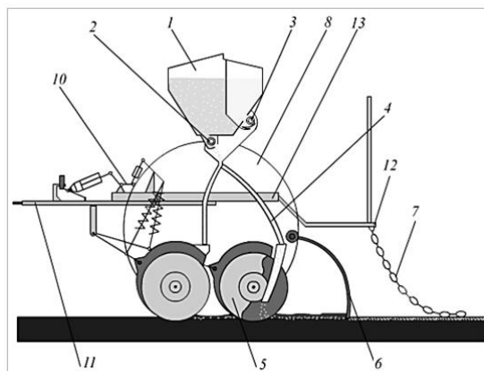
Рис. 3. Общая схема сеялки СЗ-3,6:
