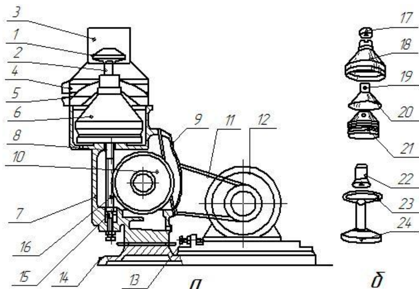
Рис. 4. Сепаратор СОМ-3-1000М:
