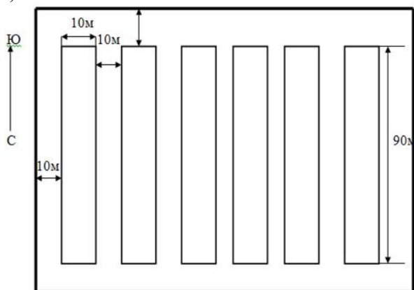
Рис. 2 План размещения токового хозяйства
