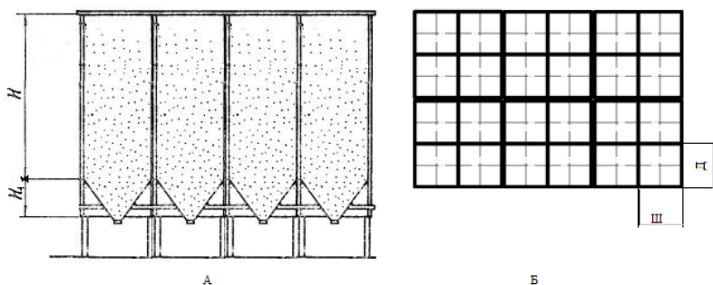
Рис. 4. Силос прямоугольного сечения: А) внешний вид, профиль: H – высота прямоугольной части силоса, H_1 – высота трапецевидной части силоса. Б) внешний вид сверху: \Pi – ширина силоса квадратного сечения, D – длинна силоса квадратного сечения
