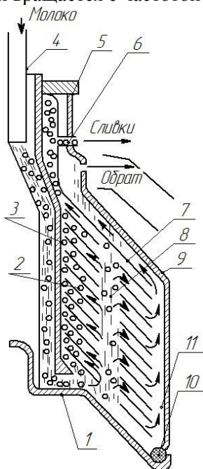
Рис. 5. Схема работы барабана сепаратора-сливкоотделителя:
