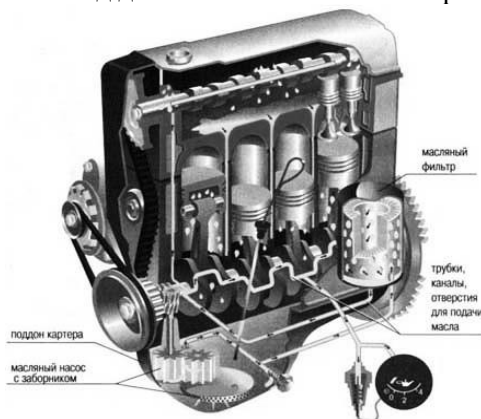
Рис. 10. Система смазки двигателя:
