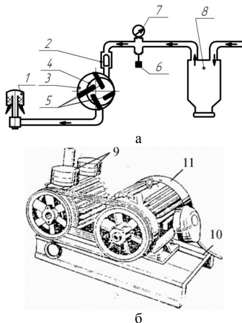
Рис. 6. Схема унифицированной вакуумной установки ВВУ-60/45:
