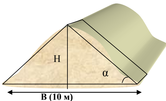
Рис. 1 Зерновой бунт удлинённой формы.
