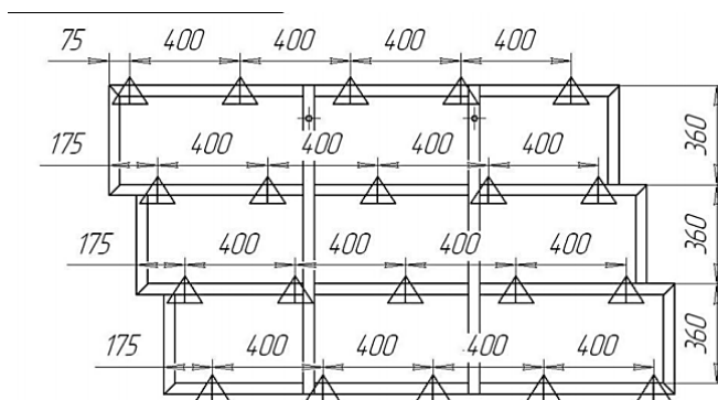
Рис. 2. Схема расстановки рабочих органов КБМ-4,2
