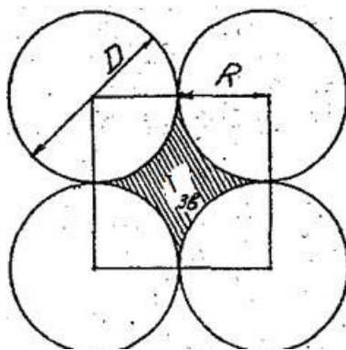
Рис. 5 Фрагмент силосного корпуса круглого сечения в разрезе:
