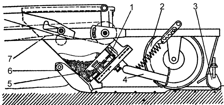
Рис. 3.23. Схема высевающего аппарата с наклонным диском: 1 – высевающий диск; 2 – прикатывающий каток; 3 – загортач; 4 – ограничитель; 5 – семенная банка; 6 – сошник; 7 – цепь центрального привода
