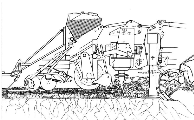
Рис. 9.14. Схема работы комбинированного агрегата серии КГ с глубококорыхлителем
