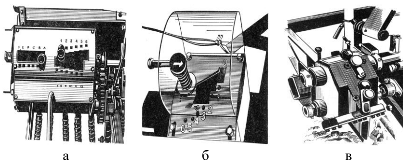
Рис. 5.2. Коробки передач привода высевальных аппаратов: а – 72-ступенчатая коробка открытого типа («Нортон») зерновой сеялки А591 «Саксония»; б – шестиступенчатая коробка передач сеялки «Моноцентра»; в – шестиступенчатая коробка передач закрытого исполнения сеялки точного высева «Аэромат» фирмы «Беккер»
