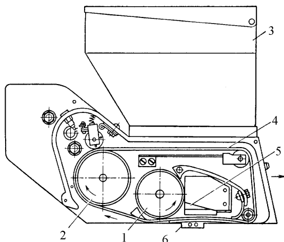
Рис. 3.28. Высеваящий аппарат сеялки «Stanhay»:
