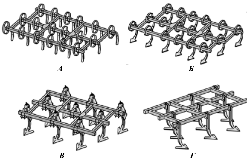
Рис. 29. Сменные модули к культиватору КБМ-4,2НУ: А – с рыхлительной лапой на подпружиненной стойке для предпосевной обработки до появления всходов сорняков; Б – со стрелчатой лапой на усиленной подпружиненной стойке для предпосевной обработки после появления всходов сорняков; В – со стрелчатой лапой на жесткой подпружиненной стойке для предпосевной обработки по стерновым фонам и обработки пара; Г – со стрелчатой лапой на жесткой стойке для обработки пара
