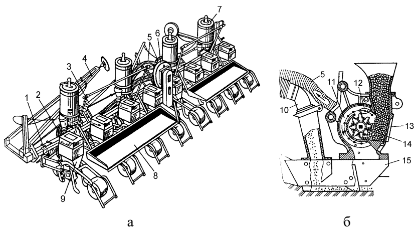
Рис. 3.16. Сеялка СУПН-8А:
