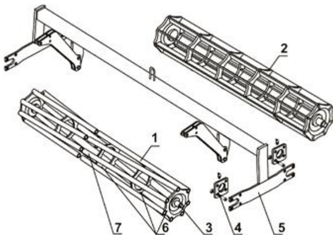
Рис. 24. Катки
