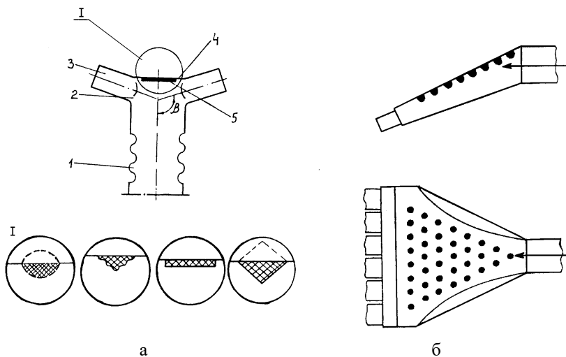
Рис. 3.13. Схемы распределительных головок высеваящих систем: а – цилиндрической: 1 – направитель; 2 – коллектор; 3 – выходные патрубки; 4 – крышка; 5 – отражатель; б – плоской
