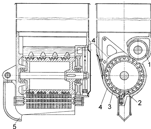
Рис. 3.31. Высевной аппарат сеялки СПП-12:
