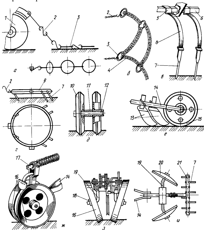
Рис. 3.8. Задельвающие устройства:
