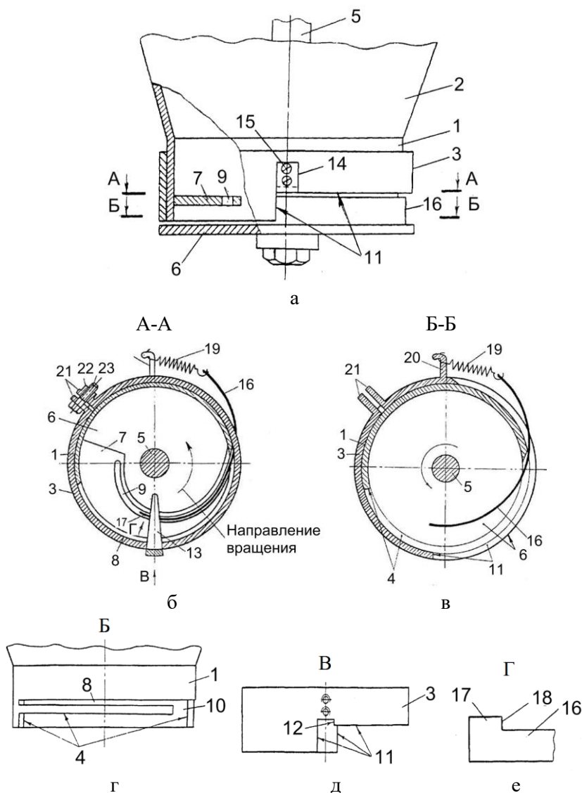
Рис. 10.6. Скребковый высевающий аппарат
