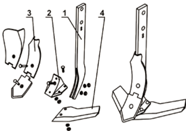
Рис. 22. Рыхлящая лапа
