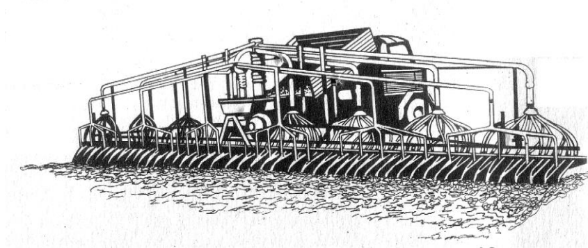
Рис. 3.3. Сеялка «Аккорд» с захватом 12 м в агрегате с тягачом «Унимог»
