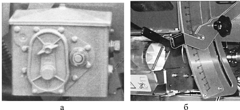
Рис. 5.3. Двухрежимная бесступенчатая коробка передач: а – общий вид коробки переада; б – рычаг и шкала бесступенчатой настройки высевающего аппарата на норму высева
