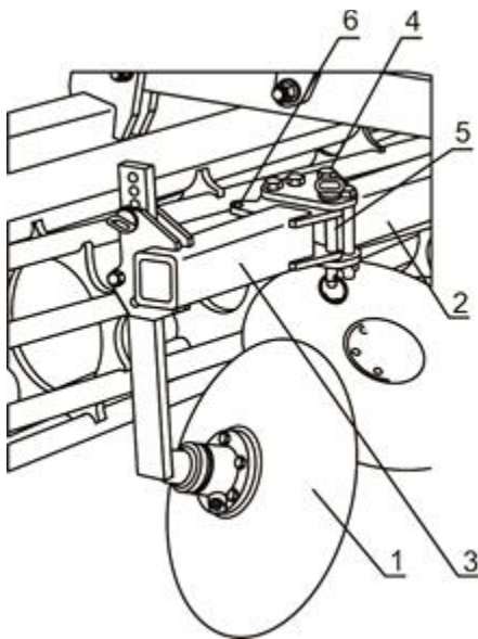
Рис. 25. Крайние диски
