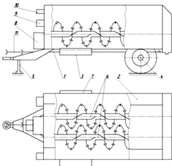
Рис. 18. Измельчитель смеситель-раздатчик кормов ИСПК-12: 1 – рама; 2 – бункер; 3 – выгрузной скребковый транспортер; 4 – ось тормозная с колесами; 5 – опора; 6 – шнеки; 7 – лоток выгрузной; 8 – масляный бак гидросистемы; 9 – дисплей весового механизма; 10 – пульт управления; 11 – карданный вал
