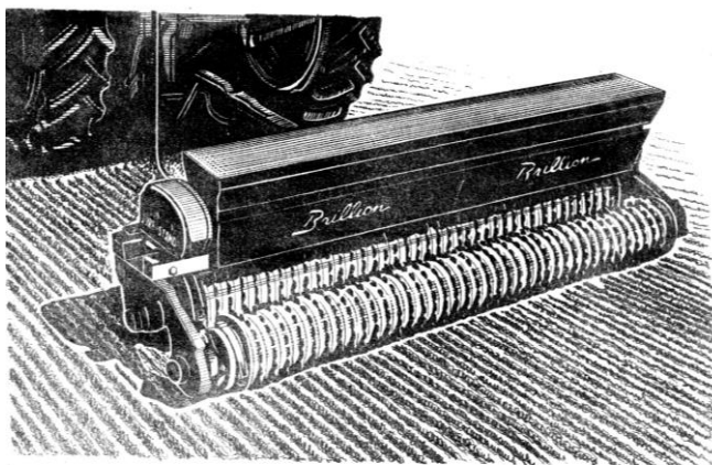
Рис. 9.17. Каток-сеялка фирмы «Бриллион»
