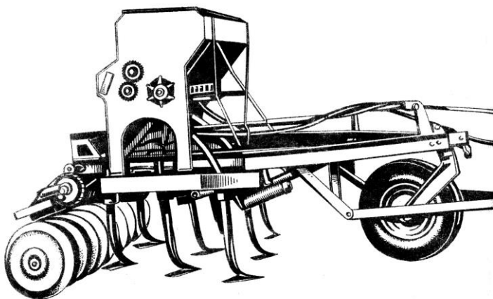
Рис. 9.16. Стерневая сеялка-культиватор СЗС-2,1
