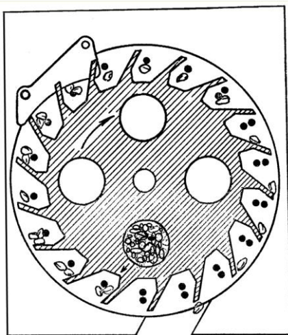
Рис. 3.38. Схема дозирования подачи семян в высевальном аппарате сеялки точного высева «Monosem»
