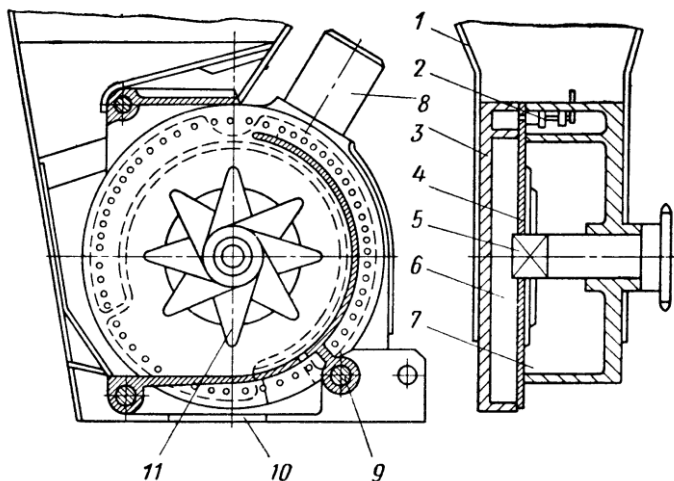
Рис. 3.36. Высевальной аппарат сеялки СПЧ-6:
