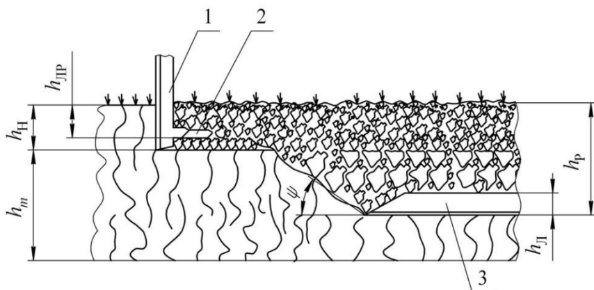
1 – нож-щелерез; 2 – лапка-рыхлитель; 3 – плоскорежущая лапа
